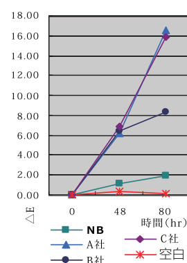
基板腐蚀测试
