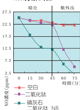
NOx分解试验
